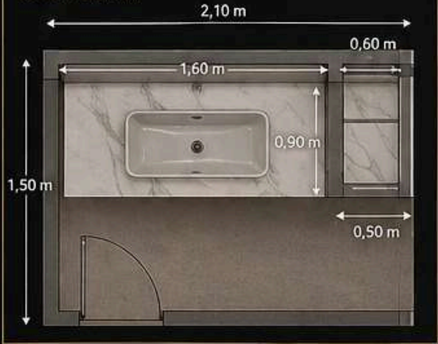
PLANTA BAIXA
