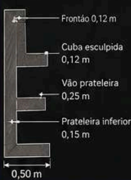
CORTE LATERAL (BANCADA)
