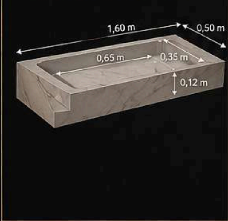
DETALHE DA BANCADA ESCULPIDA
