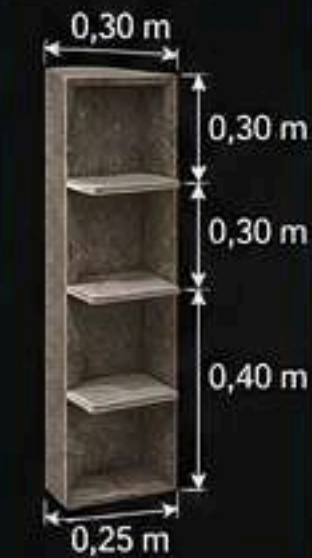
DETALHE TORRE PRATELEIRAS
