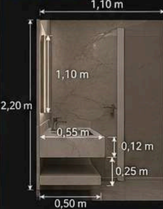
VISTA LATERAL
