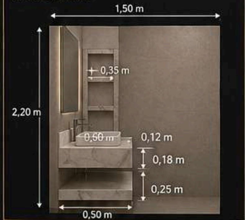
VISTA LATERAL
